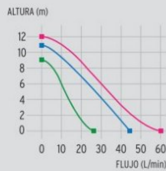
PRE-1/3 ■ Presión ajustable a 9 m ■ Presión ajustable a 11 m ■ Presión ajustable a 12 m
