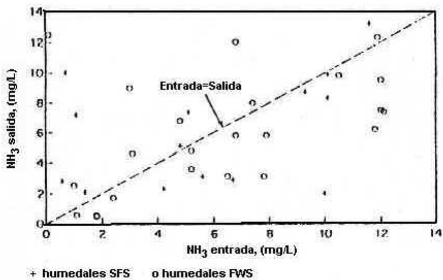
Figura 10 – Entrada de amoníaco contra salida de amoníaco en humedales artificiales.
