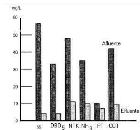
Figura 7 - Rendimientos de remoción típicos.
