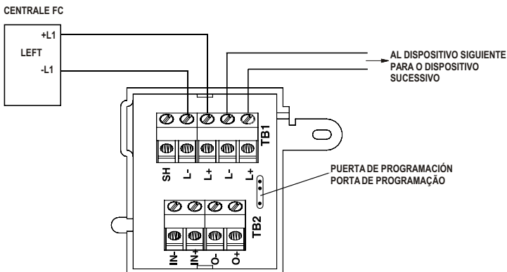
FC421CP Pulsador Externo Esquema de conexión FIG.4 FC421CP Botão para exteriores ; Esquema de conexão
