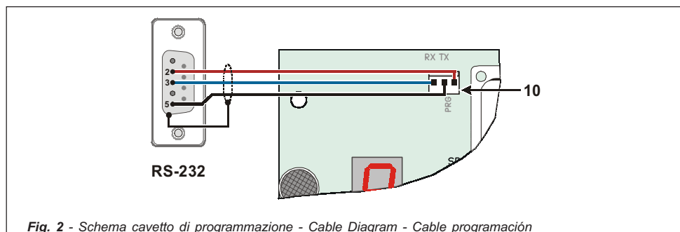
Fig. 2 - Schema cavetto di programmazione - Cable Diagram - Cable programación
