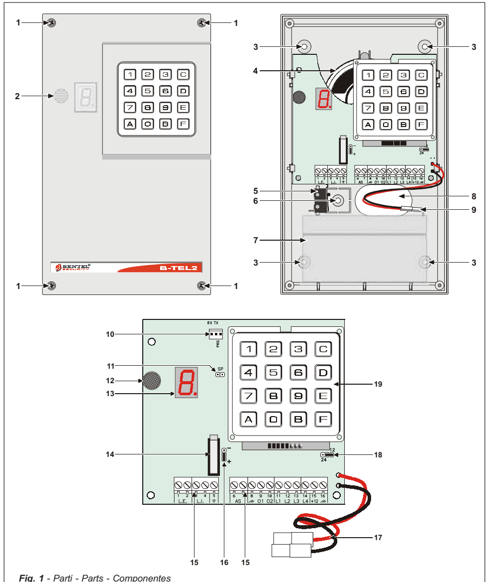
Fig. 1 - Parti - Parts - Componentes
